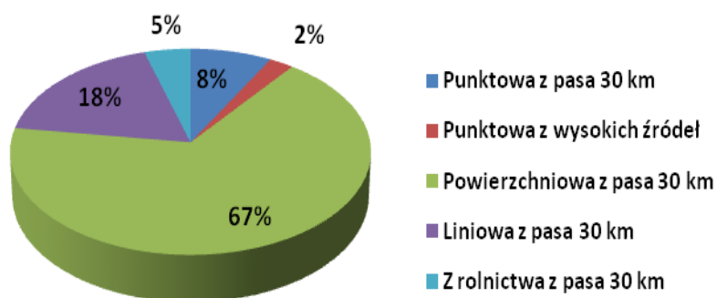
Rysunek 23 Udział procentowy emisji pyłu zawieszony PM10 poszczególnych typów poza strefą lubelską w 2015 r.
