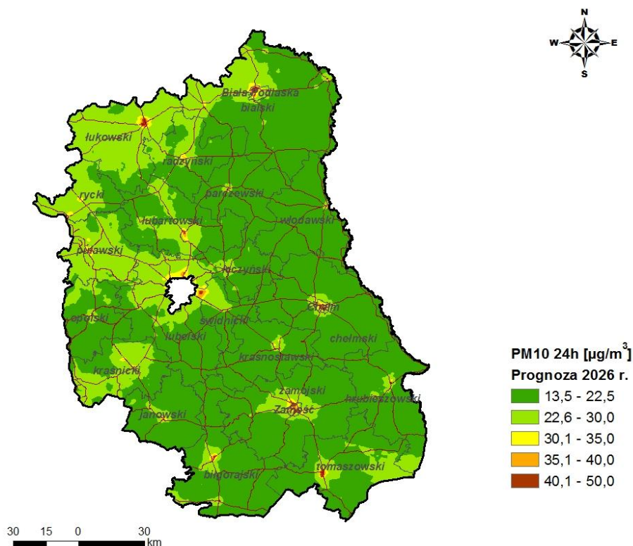
Rysunek 51 Prognozowane stężenia pyłu zawieszonego PM10 o okresie uśredniania wyników 24 h w strefie lubelskiej pochodzące z łącznej emisji wszystkich typów w 2026 r.
