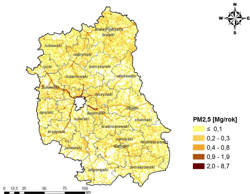
Rysunek 34 Emisja liniowa pyłu zawieszzonego PM2,5 z terenu strefy lubelskiej w 2015 r.
