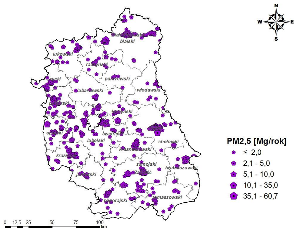
Rysunek 32 Emisja punktowa pyłu zawieszonego PM2,5 z terenu strefy lubelskiej w 2015 r.
