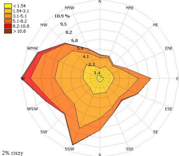
Rysunek 7 Rozkład kierunków i prędkości wiatru w wybranych miastach, wyznaczony przez model WRF/CALMET, w strefie lubelskiej w 2015 r.
