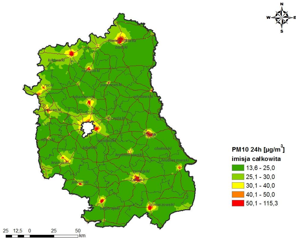
Rysunek 39 Stężenia pyłu zawieszzonego PM10 o okresie uśredniania wyników 24 h w strefie lubelskiej pochodzące z łącznej emisji wszystkich typów w 2015 r.
