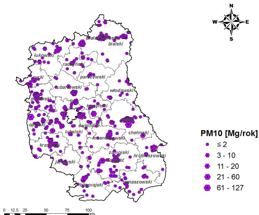
Rysunek 25 Emisja punktowa pyłu zawieszonego PM10 z terenu strefy lubelskiej w 2015 r.
