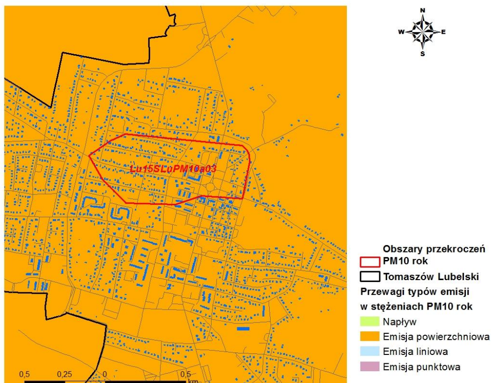
Rysunek 48 Przewagi typów emisji w stężeniach pyłu zawieszonego PM10 rok w obszarach przekroczeń w Tomaszowie Lubelskim w 2015 r.
