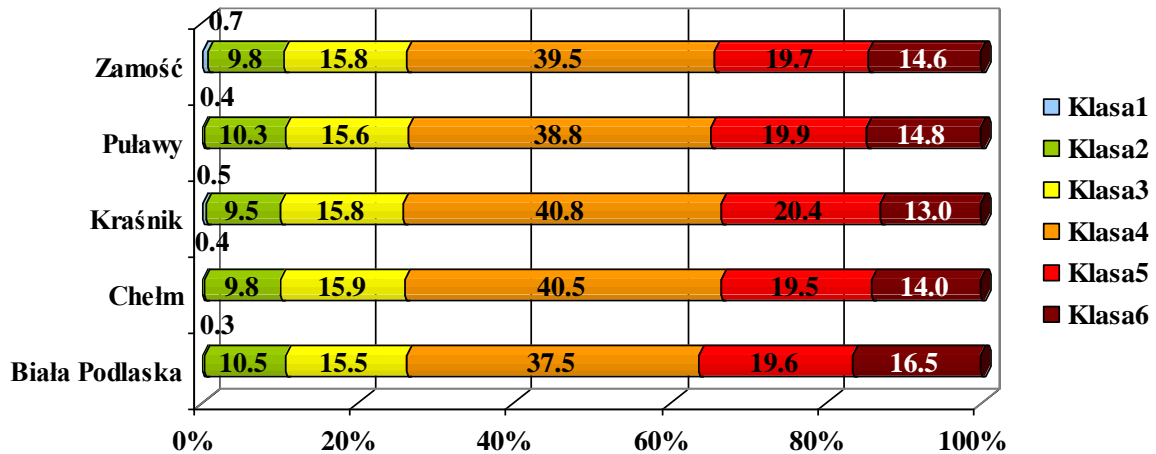
Rysunek 15 Rozkłady prawdopodobieństwa występowania klas równowagi atmosfery wyznaczone przez model WRF/CALMET w strefie lubelskiej w 2015 r.
