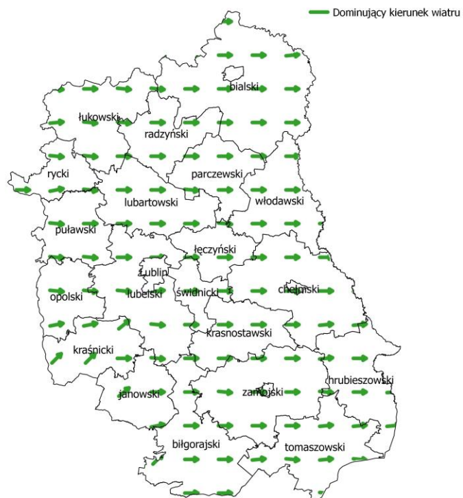
Rysunek 6 Dominujący (w roku) kierunek wiatru wyznaczony przez model WRF/CALMET w strefie lubelskiej w 2015 r.
