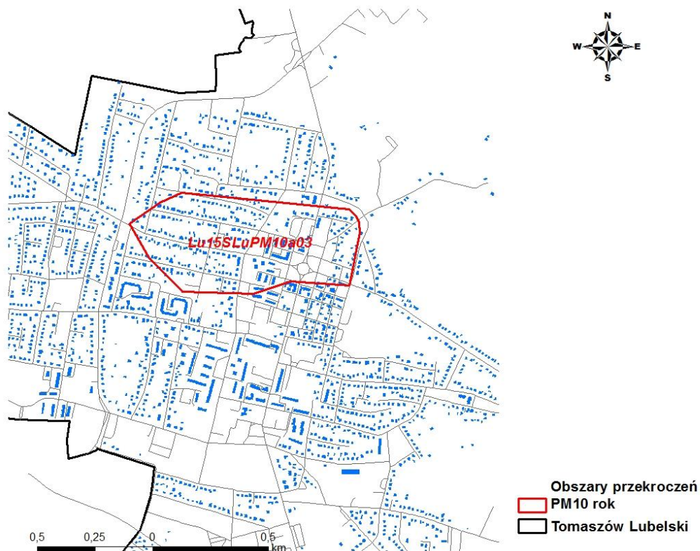
Rysunek 47 Obszar przekroczeń poziomu dopuszczalnego pyłu zawieszonego PM10 rok w Tomaszowie Lubelskim w 2015 r.
