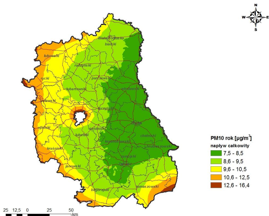
Rysunek 38 Stężenia pyłu zawieszonego PM10 o okresie uśredniania wyników rok w strefie lubelskiej pochodzące z tła całkowitego w 2015 r.
