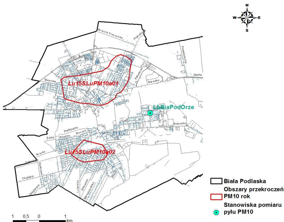
Rysunek 45 Obszary przekroczeń poziomu dopuszczalnego pyłu zawieszonego PM10 rok w Białce Podlaskiej w 2015 r.
