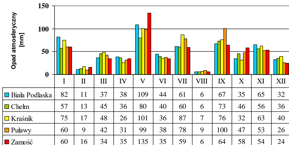
Rysunek 11 Rozkłady miesięcznych sum opadów atmosferycznych wyznaczone przez model WRF/CALMET w strefie lubelskiej w 2015 r.
