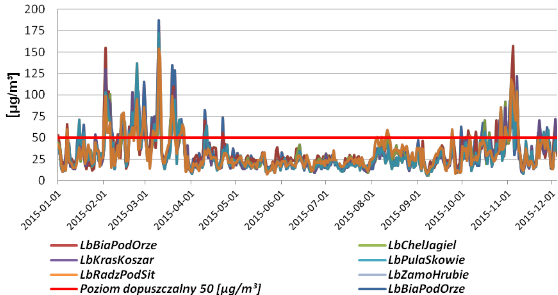
Rysunek 18 Roczny przebieg średnich dobowych wartości pyłu zawieszonego PM10 na stanowiskach pomiarowych w strefie lubelskiej w 2015 r.
