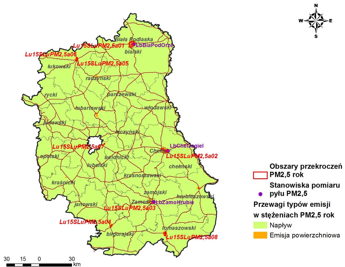
Rysunek 50 Przewagi typów emisji w stężeniach pyłu zawieszonego PM2,5 rok w obszarach przekroczeń w północnej części strefy lubelskiej w 2015 r.
