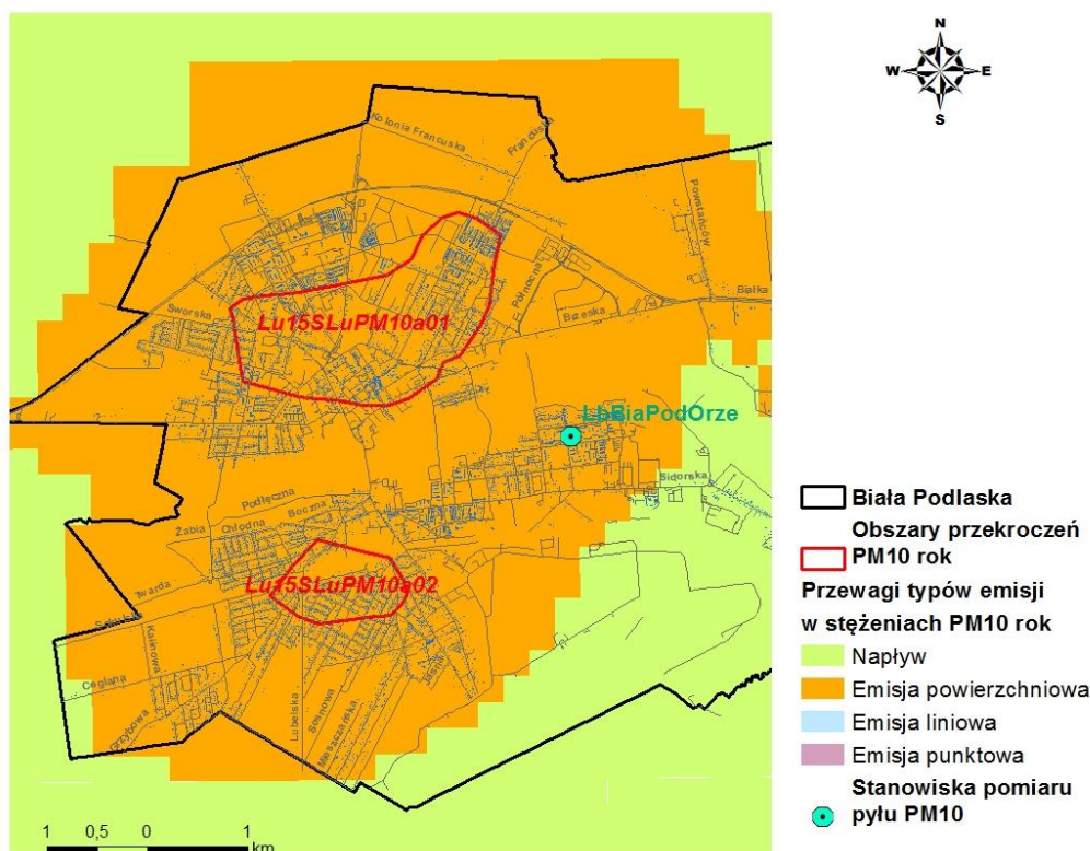
Rysunek 46 Przewagi typów emisji w stężeniach pyłu zawieszonego PM10 rok w obszarach przekroczeń w Białce Podlaskiej w 2015 r.
